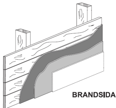
Figur 5: Illustration av en enklare icke bärande konstruktion av brandvägg kan se ut. Brandklass EI-60. (Källa: LBK, 2009)
