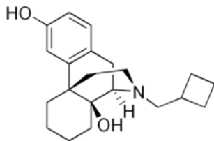
Figur 3. Butorfanol struktur (från www.wikipedia.org )
