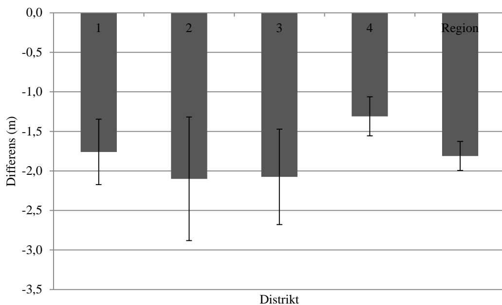
Figur 5. Genomsnittlig differens mellan angiven övre höjd (m) i trakt direktiv och i den objektiva inventeringen, uppdelat per distrikt. Felstaplarna anger den skattade differensens medelfel. Värderna saknas för distrikt 5.
