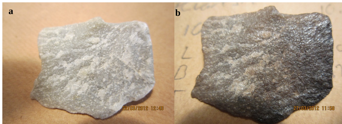
Figur 17a. Kvartsit., försök 1b, djup-1, före bränning. Figur 17b. Kvartsit, försök 1b, djup -1 efter bränning. Figure 17a. Quartzite, replicate 1b, depth -1, pre-burn. Figure 17b. Quartzite. Replicate 1b, depth -1, after burning.
