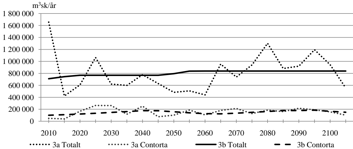
Figur 7. Årlig avverkad volym med möjlighet att välja gallring (strategi 3), totalt och contorta. Med (strategi 3b) och utan (strategi 3a) jämnhetskrav. Figure 7. Annual harvested volume with the opportunity to thin (strategy 3), total volume and volume of Lodgepole pine. With (strategy 3b) and without (strategy 3a) even-flow restrictions.
