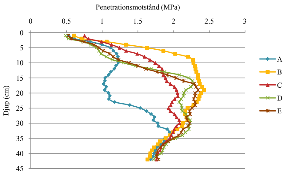
Figur 23. Penetrometermotstånd i försök L2-4049. Linjerna visar A=Plöjning, B=Carrier 2ggr, C=Direktsådd, D=Topdown djup, E=Kultivator 2ggr
