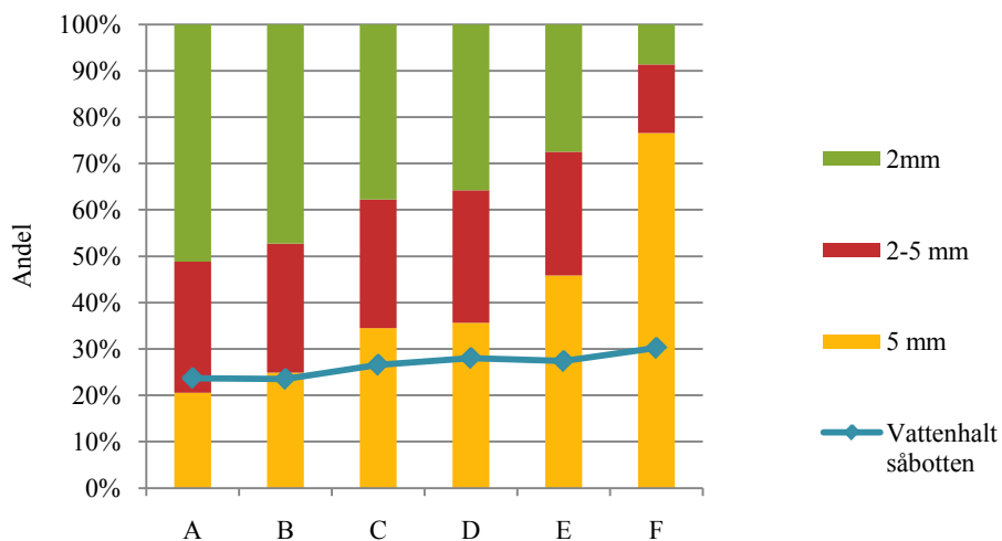
Figur 14. Aggregatstorleksfördelning i såbädd och vattenhalt i såbotten hos R2-4140 Vreta Kloster. Staplarna visar A=Plöjning 23 cm, B=Grund plöjning 12 cm, C=Kultivering 10-12 cm, D=Djupkultivering 20 cm, E=Carrier 5 cm, F=Direktsådd
