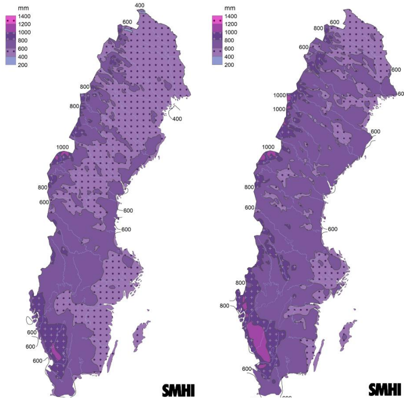
Figur 24. Kartor från SMHI som visar den normala årsnederbörden (mm) under perioden 1960–1990 (vänster), och under perioden 1991–2020 (höger).
