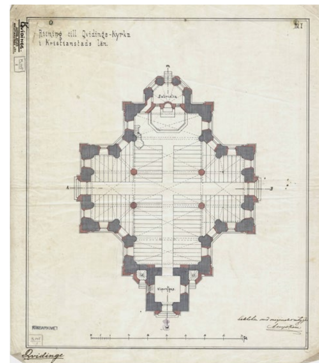
(Figur 19) Planritning av Kvidinge kyrka
