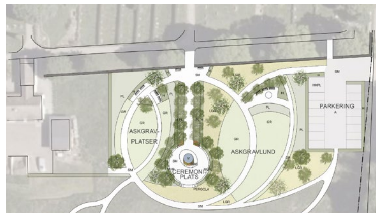
(Figur 33) Plan på Ceremoniplats - Enslöv kyrkogård
