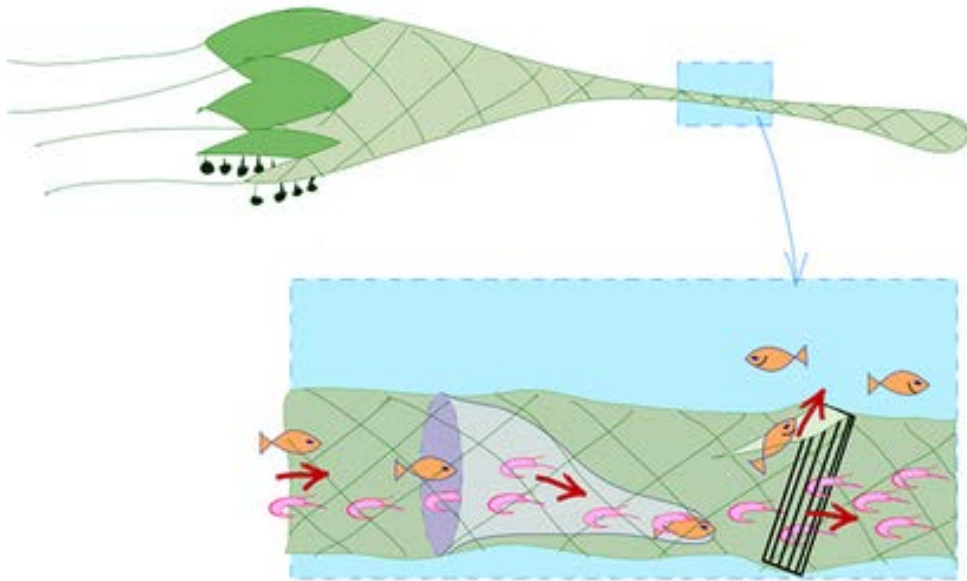
Figur 1. Schematisk bild över Kostertrålen. Källa: Samförvaltning norra Bohuslän, [hämtad 2022-04-25.], http://samforvaltningnorrabohuslan.se/projekt.html (egen bearbetning)
