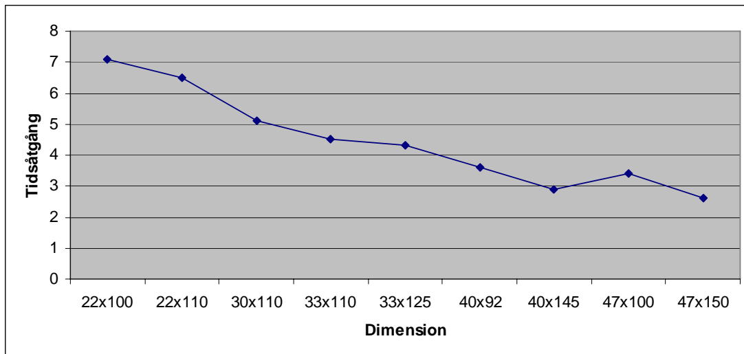
Figur 6. Tidsåtgång per m 3 hyvlat för olika dimensioner.
