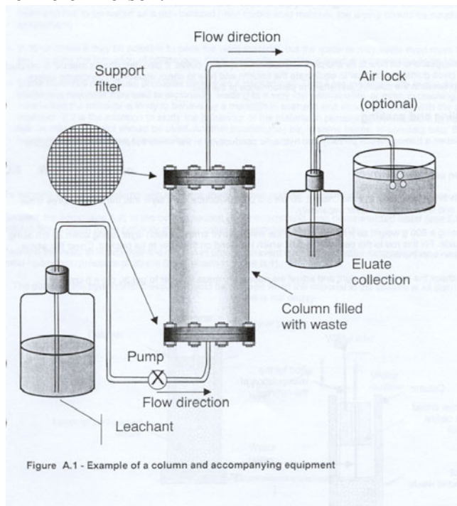
Figur 7: Illustration över kolonnen och övrigt material som används vid kolonnstest
