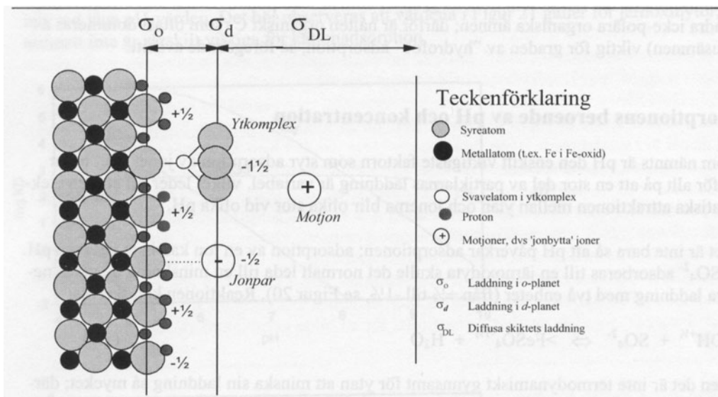
Figur 3: I figuren visas jonbyte och ytkomplexbindning till en oxidtyta. Eftersom den sammantagna laddningen på oxidtytan (tillsammans med jonparet och ytkomplexet) blir -1 , befinner sig en envärd katjon i det diffusa skiktet (Gustafsson m.fl. 2003a).
