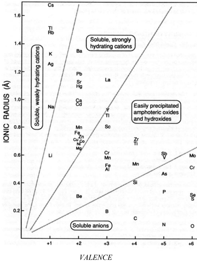
Figur 5: Oorganiska ämnens löslighet varierar med jonradien (ionic radius) och dess oxidationstal (valence).
