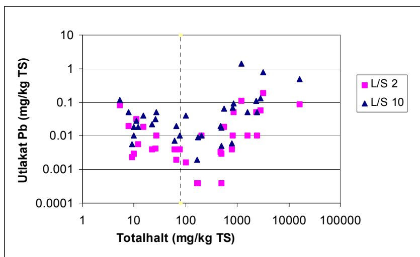
Figur 13: Koncentration utlakad Pb vid L/S 2 och L/S 10 mot totalhalten, den streckade linjen motsvarar Naturvårdsverkets generella riktvärde för KM
