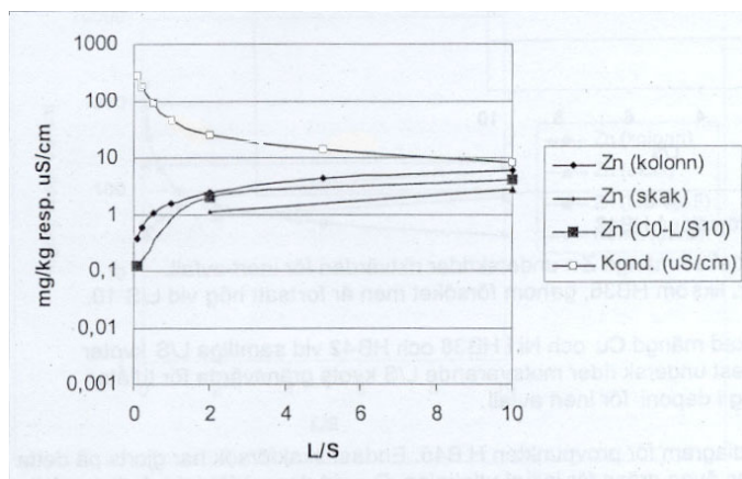
Figur 8: Kolonntest, skaktest och konduktivitet för zink (Danske GeoservEx A/S, 2003).
