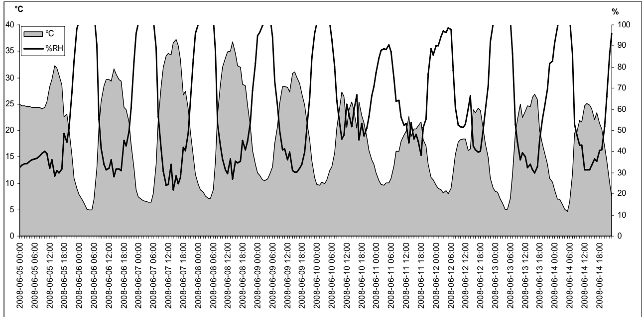
Figur 3. Lufttemperaturer och relativa luftfuktighet under en åttadagsperiod i juni 2008. Värdena kommer från en plasttunnel i Skåne (Svensson, 2009). Att den relativa luftfuktigheten är över 100 % antas bero på att givarna blivit för blöta och överreagerat.
