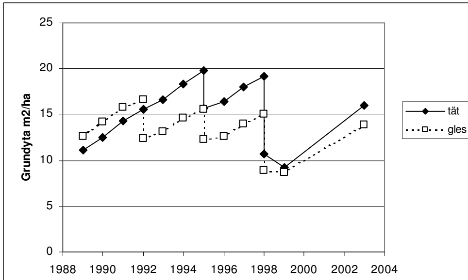
Figur 1. Tätheten (grundytan, m 2 /ha) i glesa och täta skärmen i Vedby 1989 till 2003. Figur 1. Density (basal area, m 2 /ha) in the normal and dense shelter wood, 1989 to 2003
