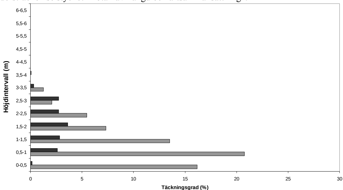
Figur 15a. Medelvärden för täckningsgraden av de överlevande lavarna på samtliga undersökta trädets stötsida. Svart stapel brända träd och grå stapel kontrollträd.
