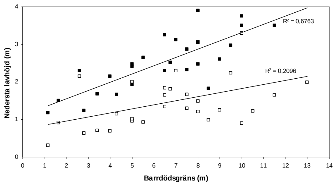
Figur 5. Sambandet mellan barrdödsgräns i tallar och höjden för nedersta överlevande lavbål. Linjära trendlinjer är utsatta för respektive sida. Trädets stötsida ( \square ) respektive läsida ( \blacksquare ).
