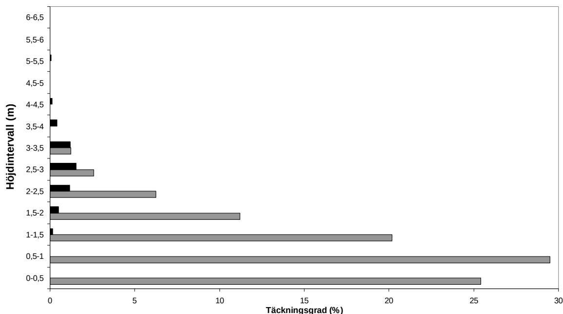
Figur 15b. Medelvärden för täckningsgraden av de överlevande lavarna på samtliga undersökta trädets läsida. Svart stapel brända träd och grå stapel kontrollträd.
