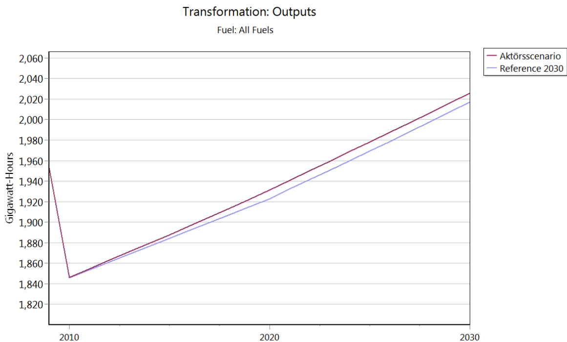
Figur 12. Levererad elektricitet
